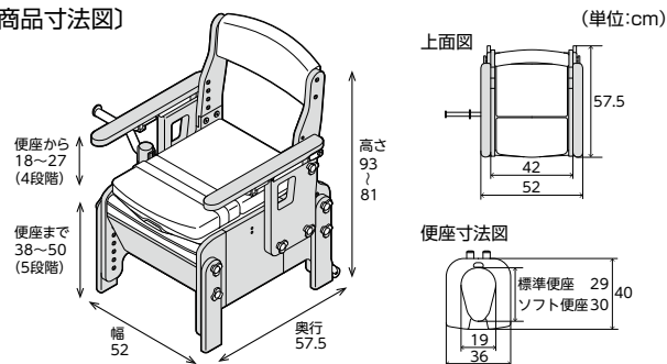
〔商品寸法図〕
