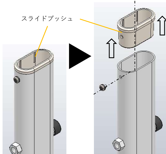
内支柱を引き抜いた後の外支柱
