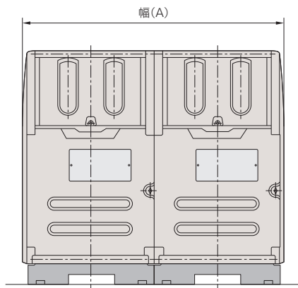
#300 連結仕様 固定台
