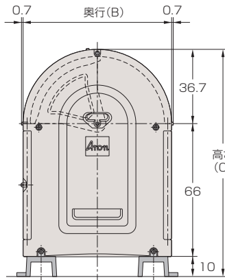
#500 連結仕様 固定台
